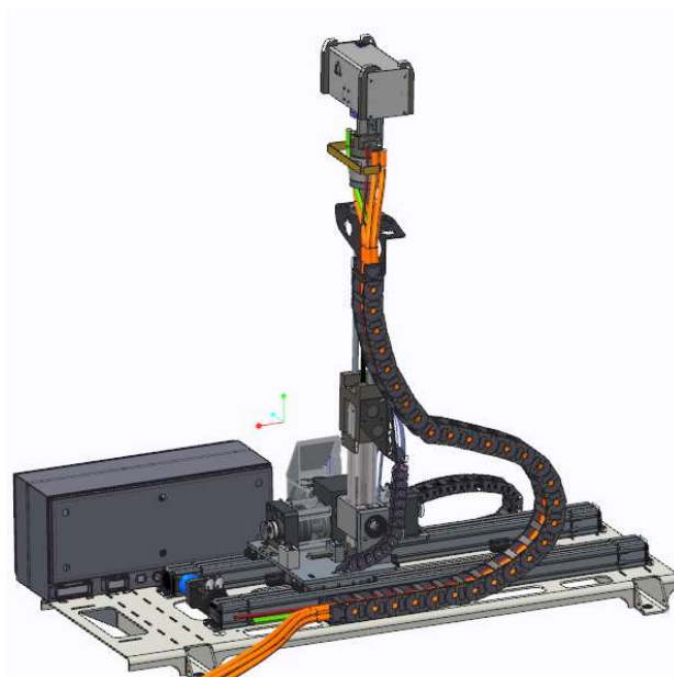
Figura 5 - ETS in posizione alta (corsa al 100%)
